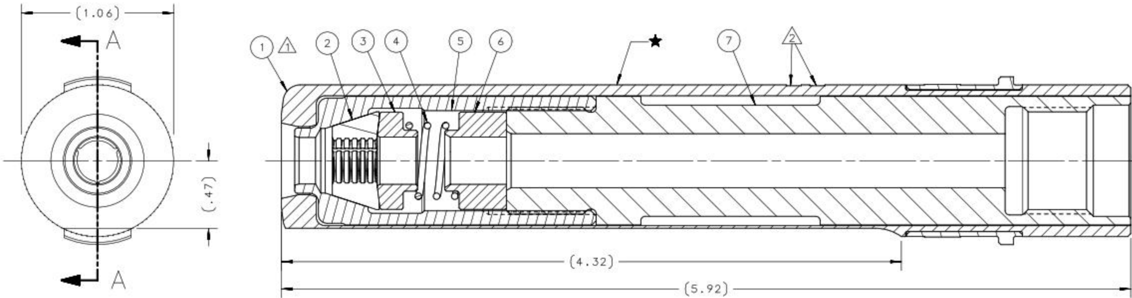
SECTION A-A
