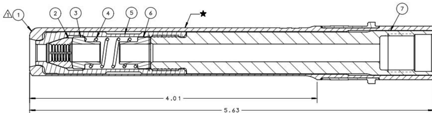
SECTION A-A
