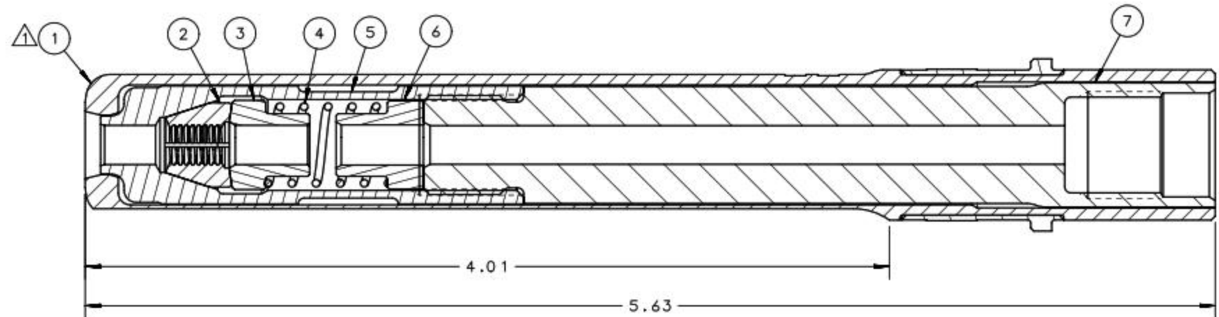
SECTION A-A
