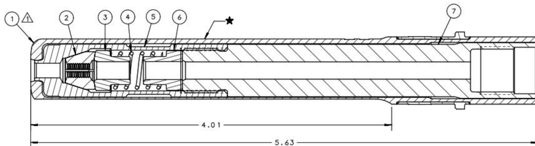
SECTION A-A
