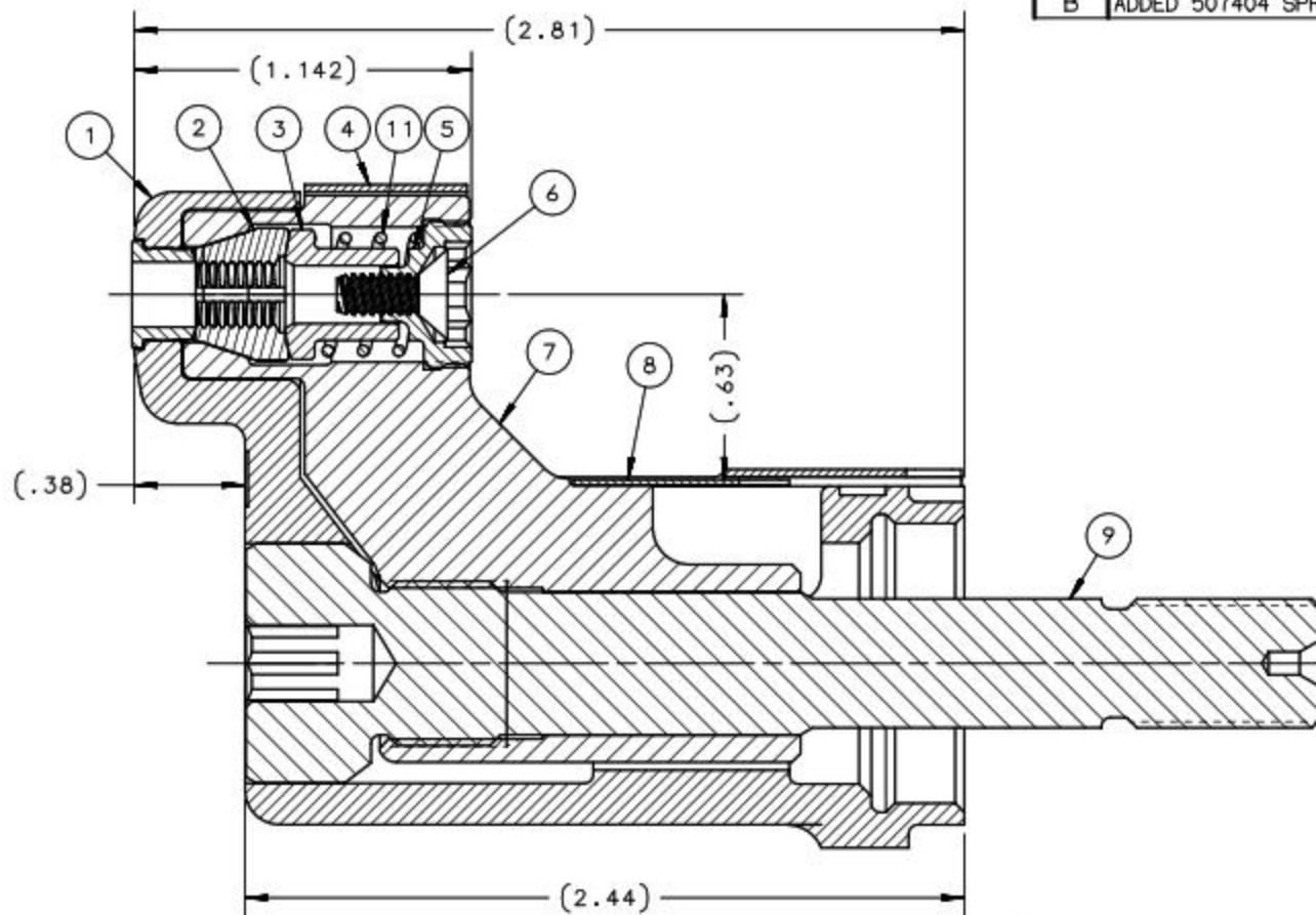
SECTION A-A
