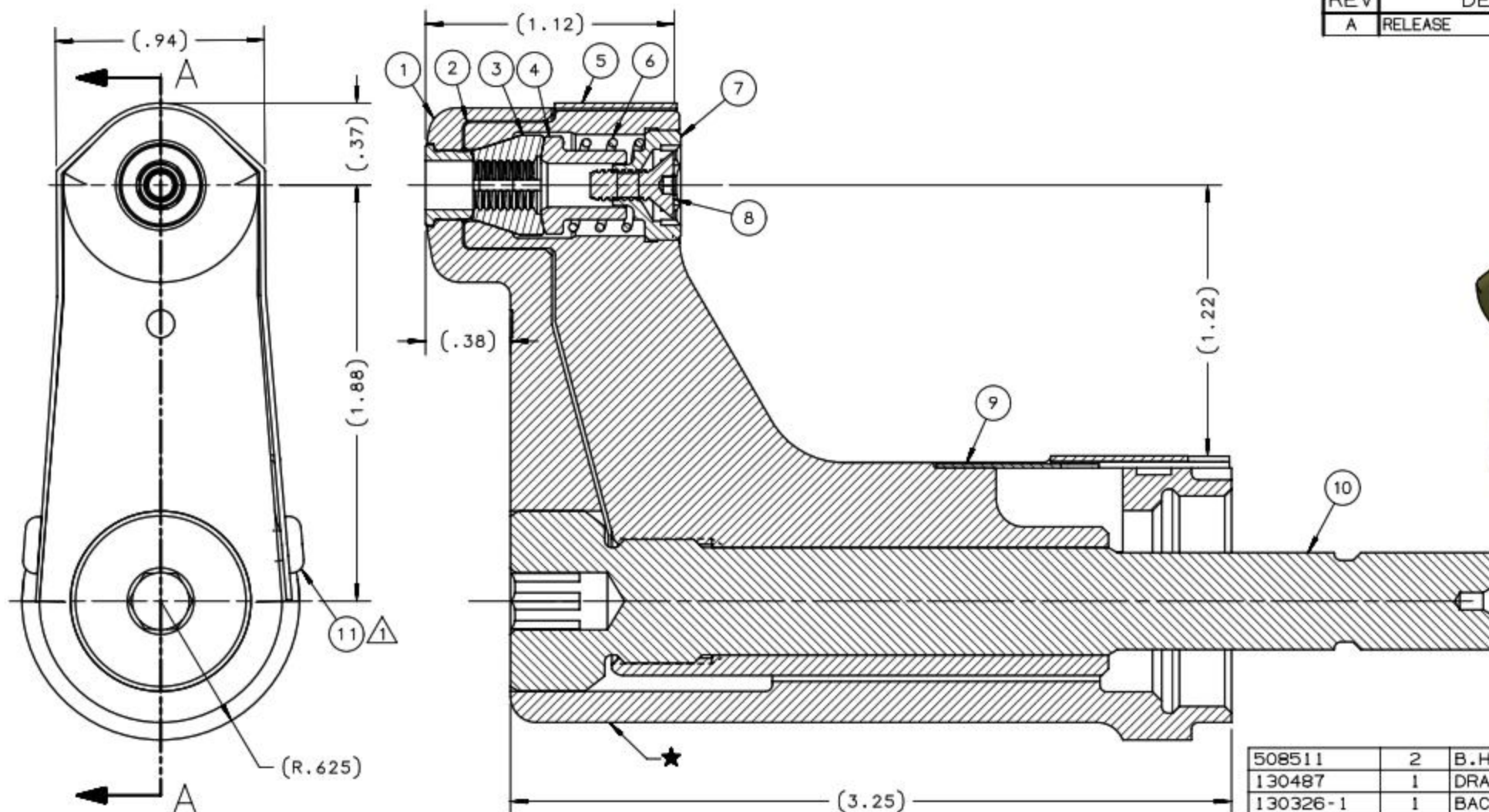
SECTION A-A
