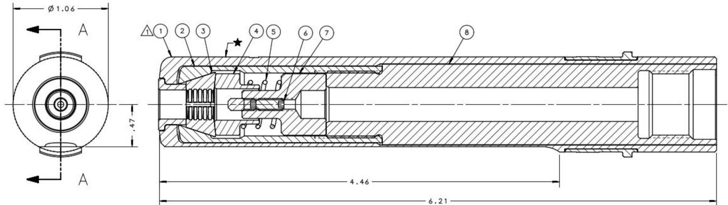
SECTION A-A
