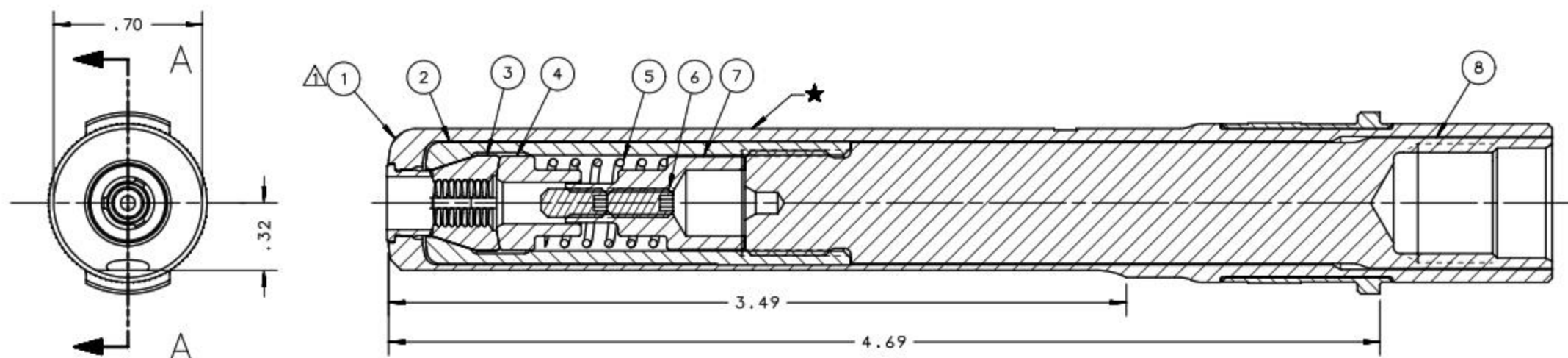
SECTION A-A
