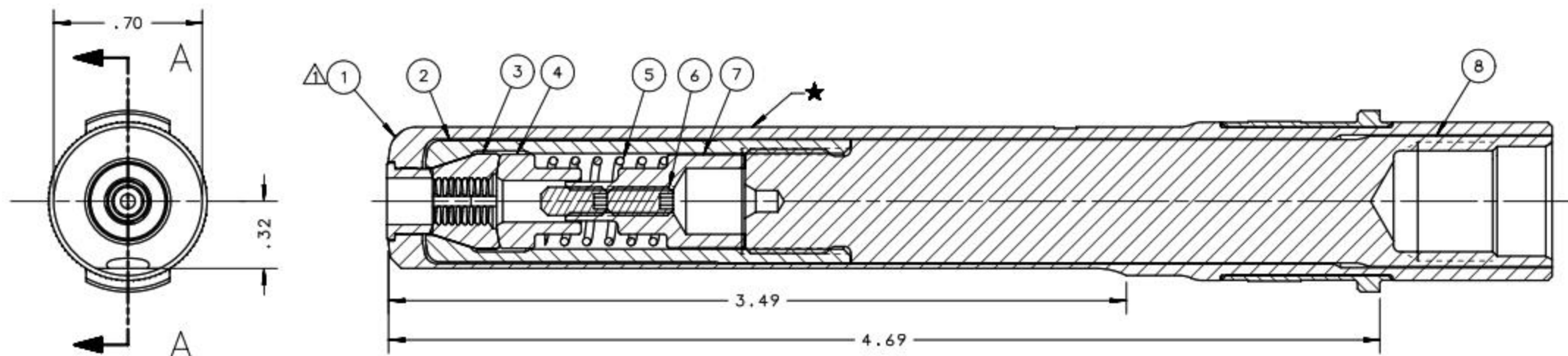
SECTION A-A
