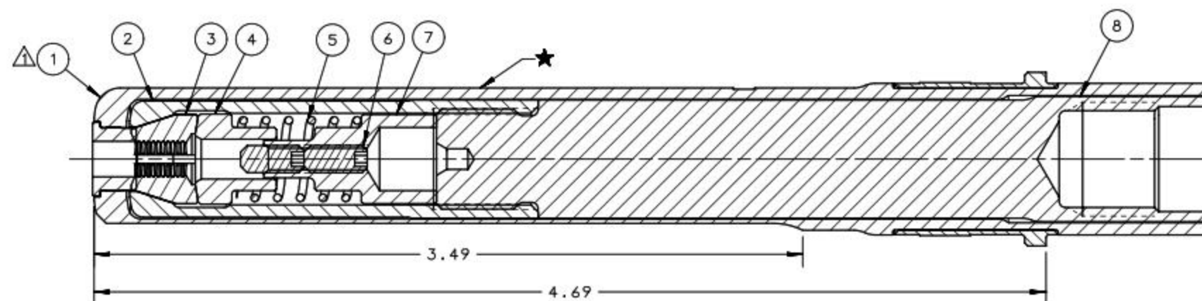
SECTION A-A
