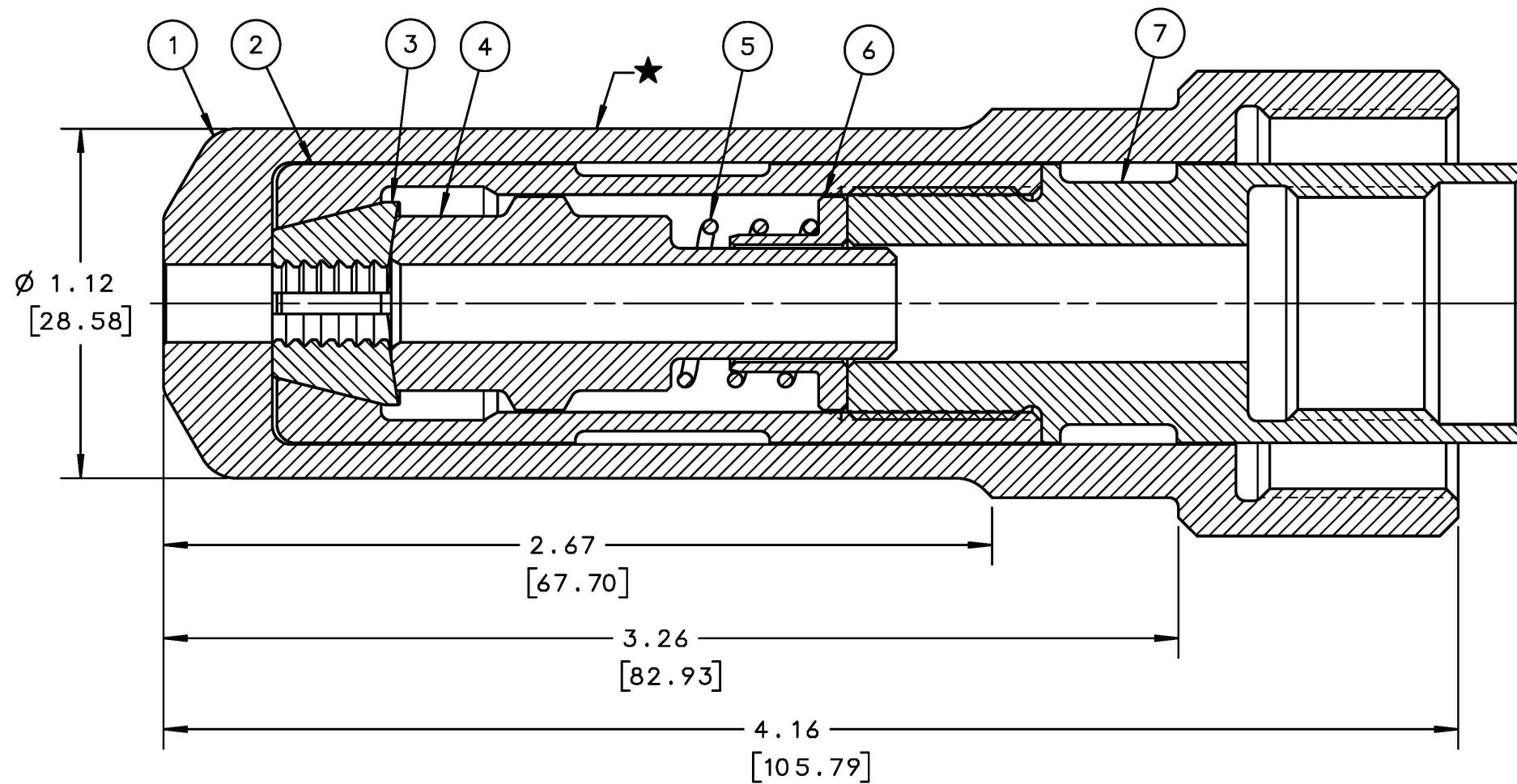
SECTION A-A
