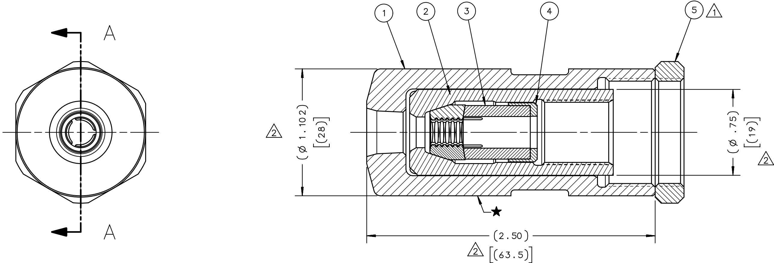
SECTION A-A
