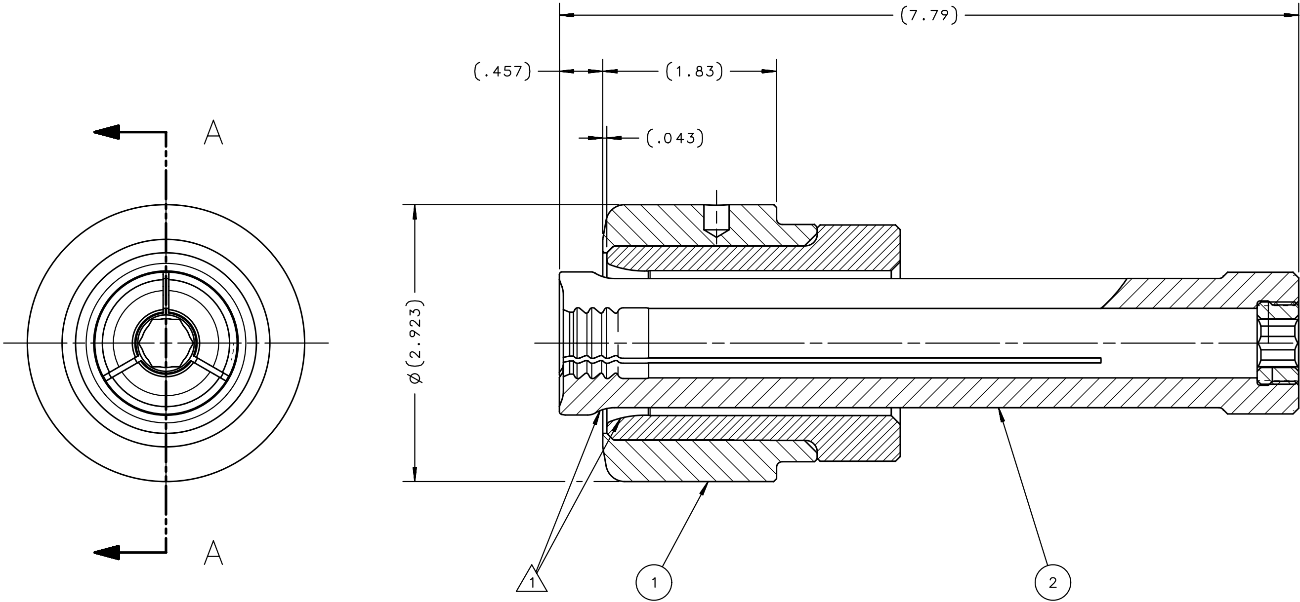
SECTION A-A
