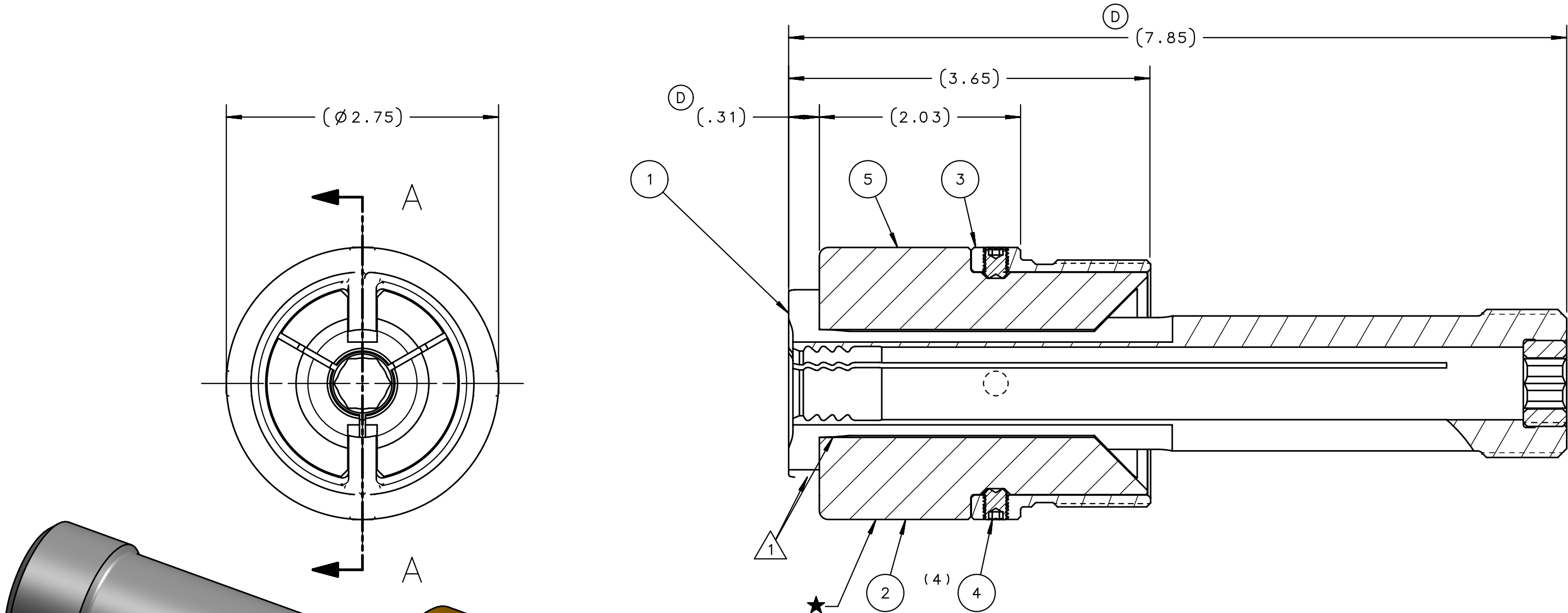
SECTION A-A
