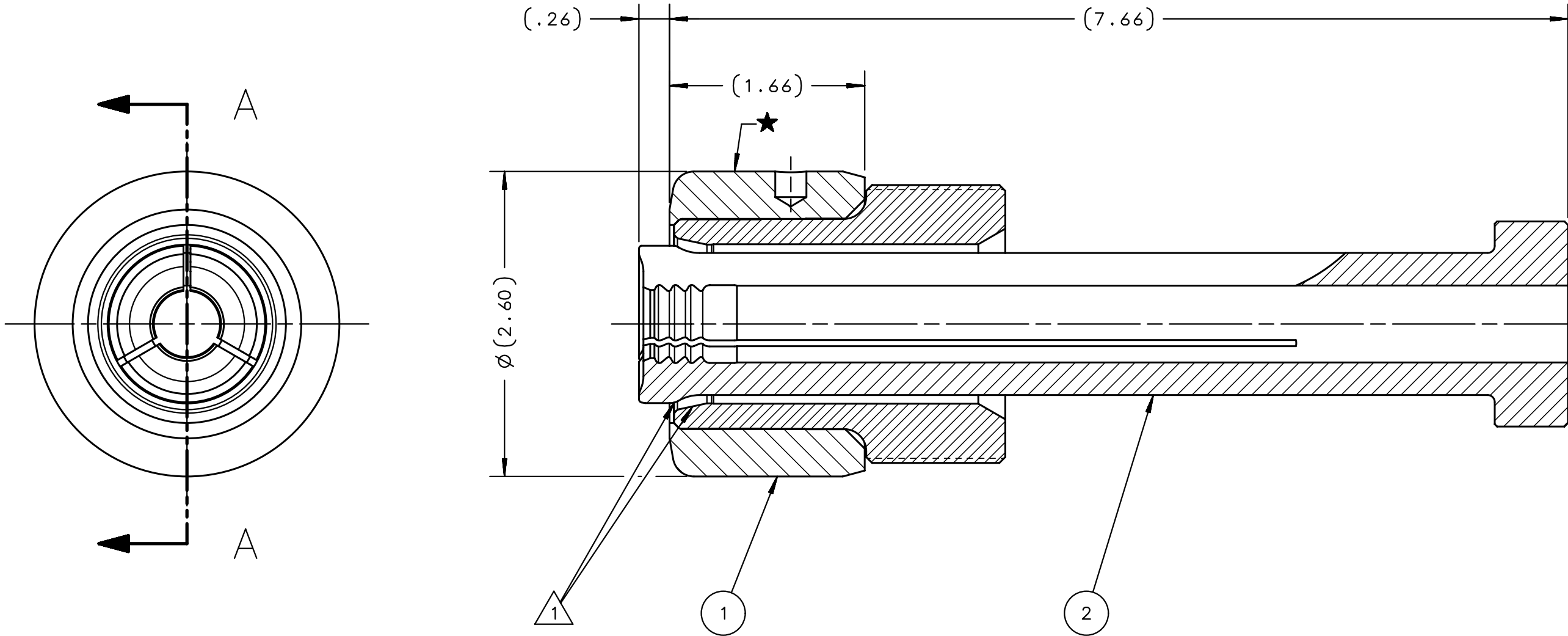
SECTION A-A
