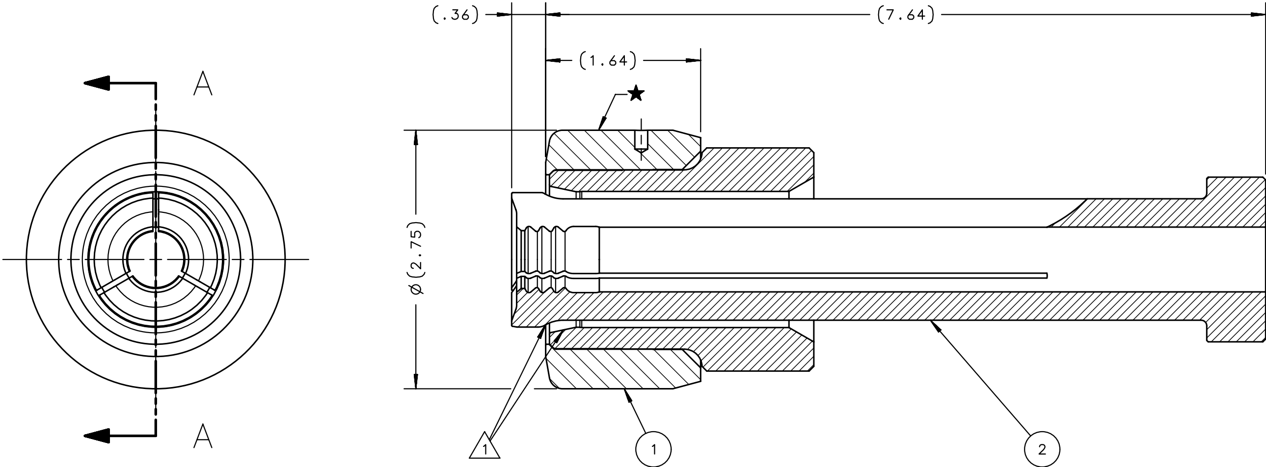
SECTION A-A
