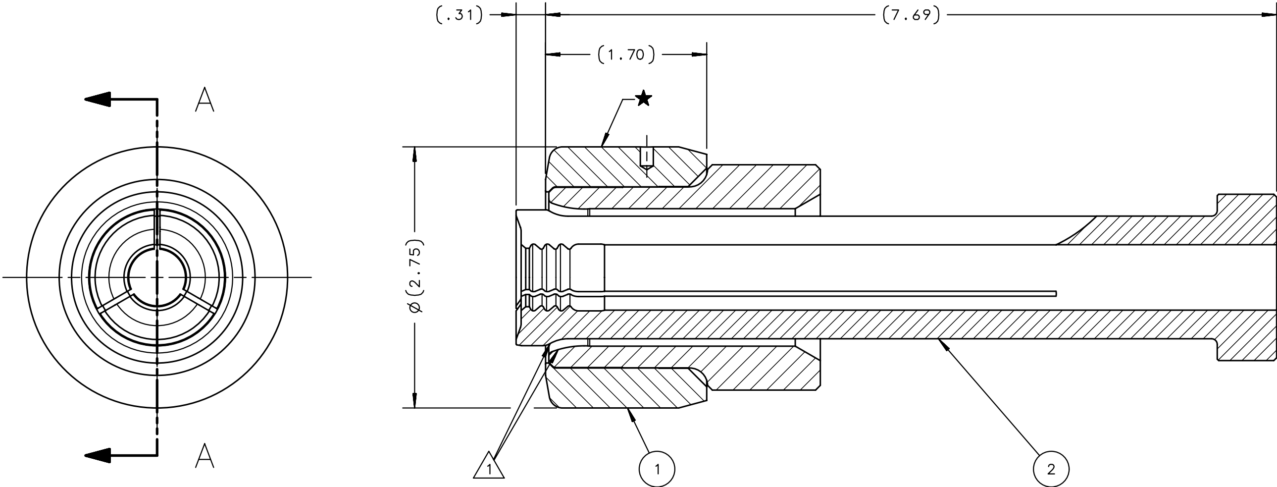
SECTION A-A
