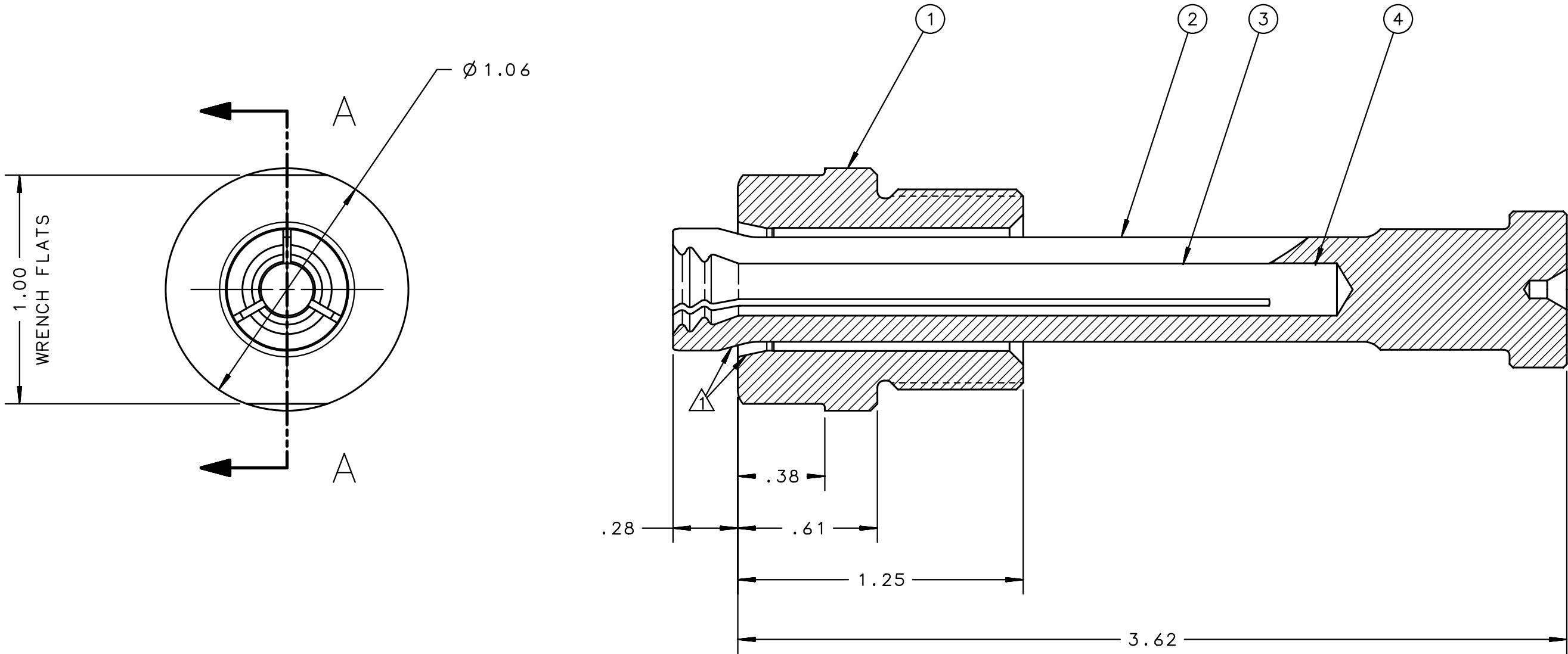
SECTION A-A
