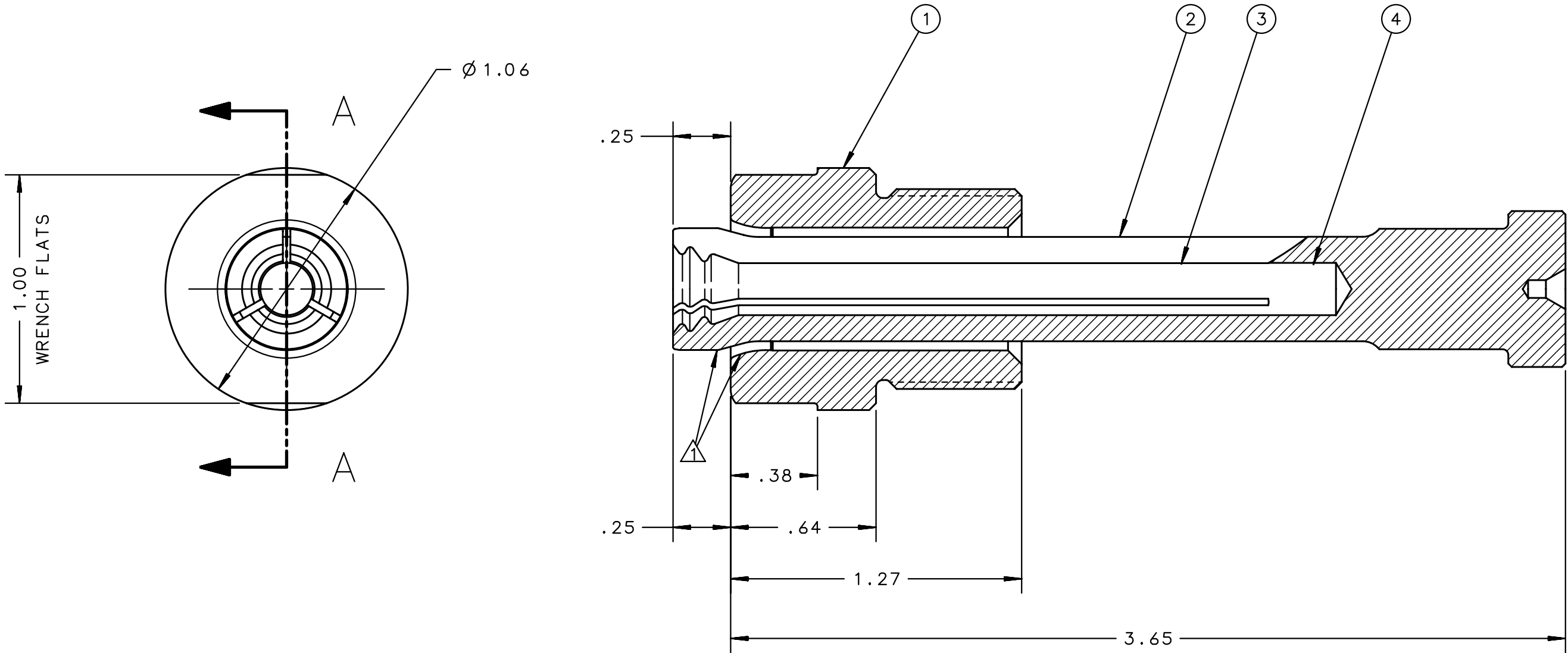
SECTION A-A
