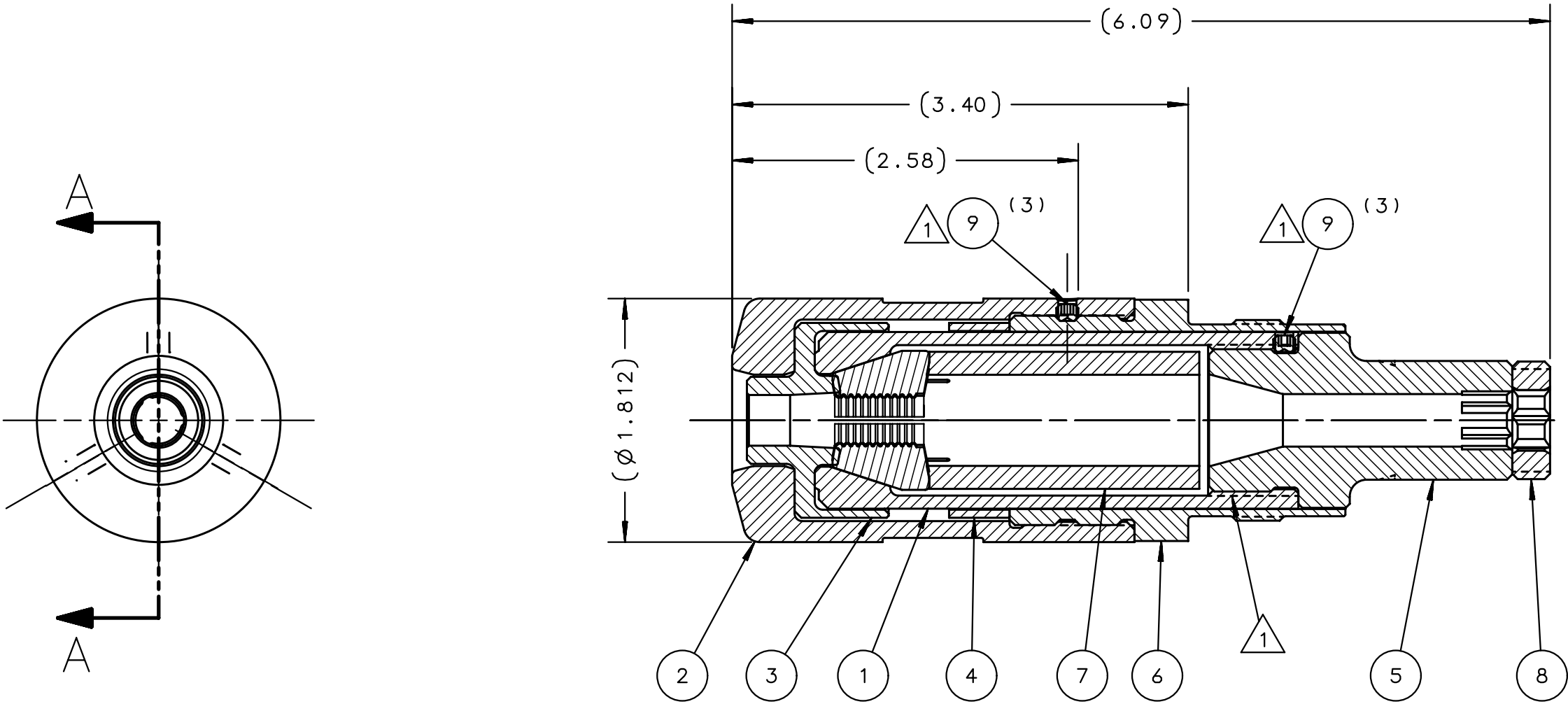
SECTION A-A
