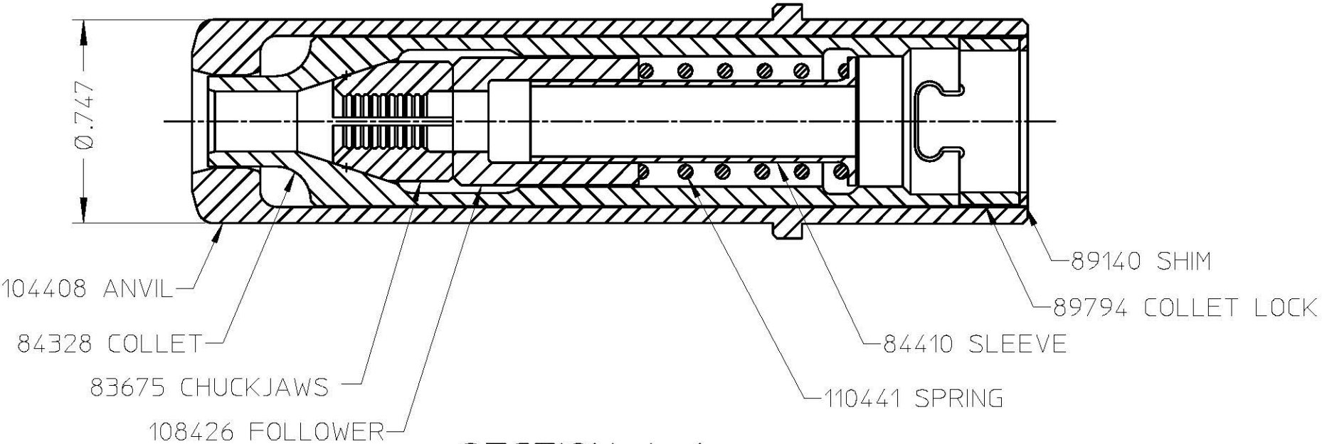
SECTION A-A
