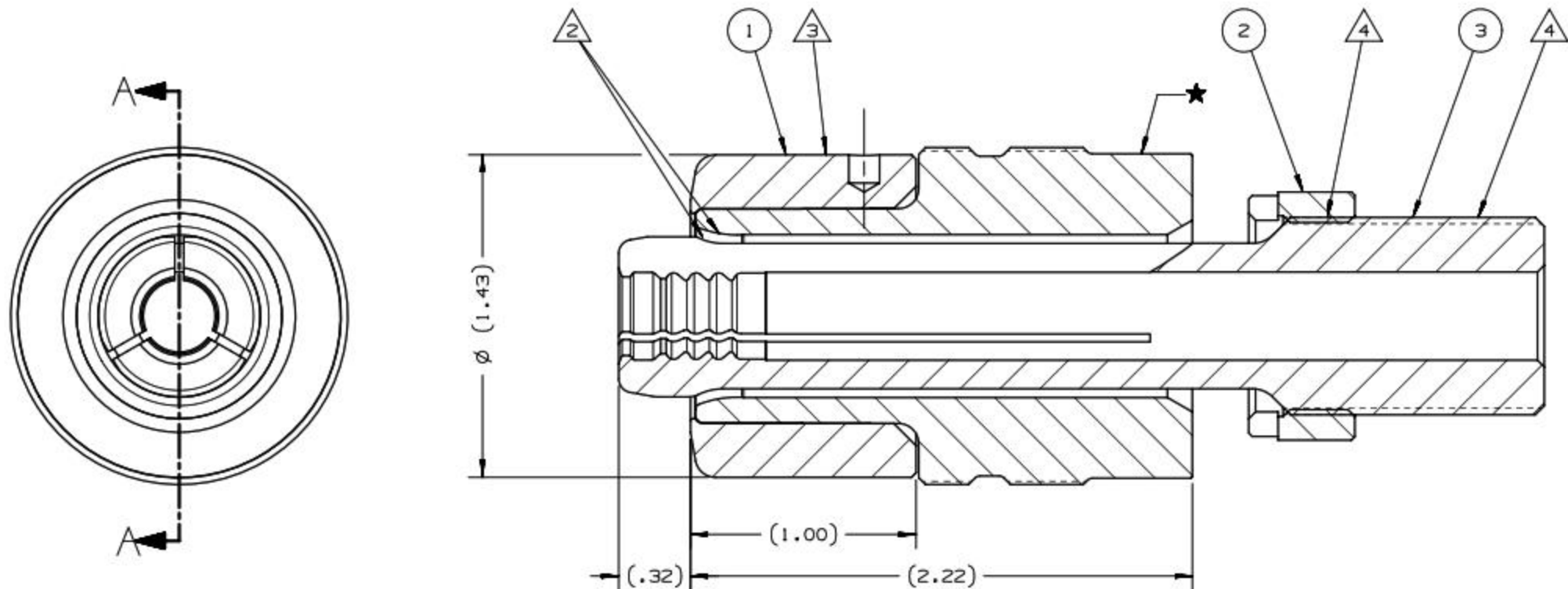
SECTION A-A
