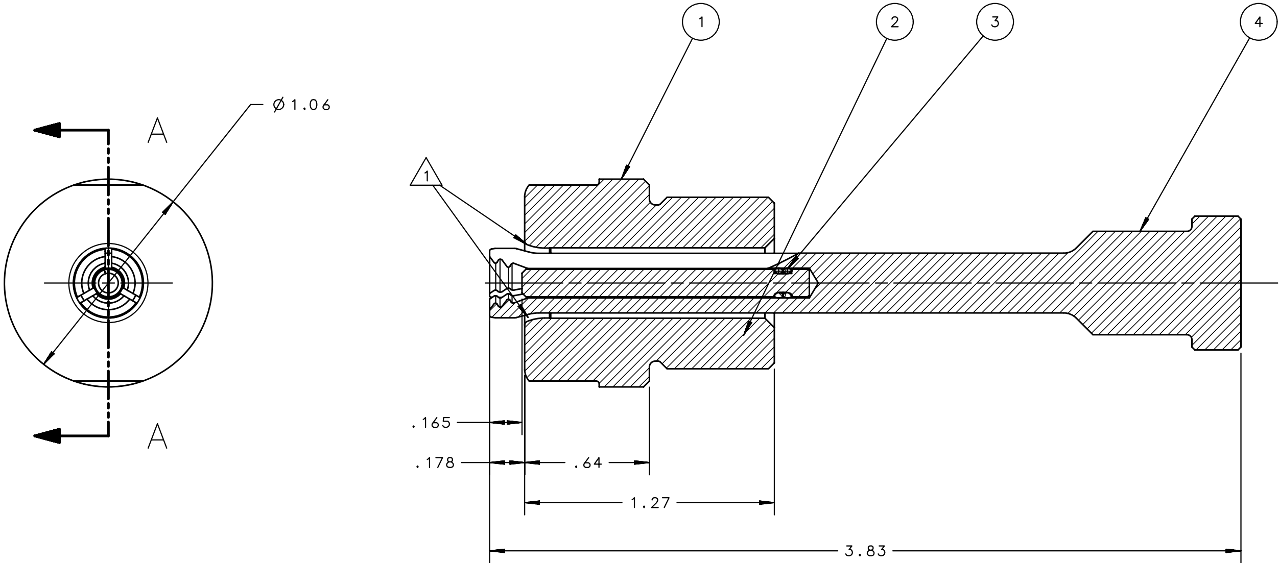
SECTION A-A
