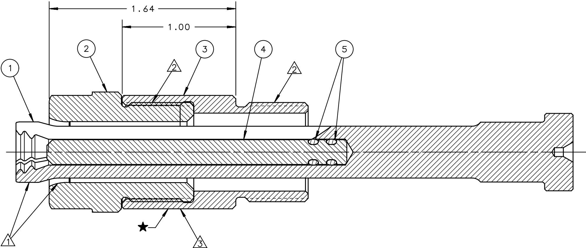
SECTION A-A
