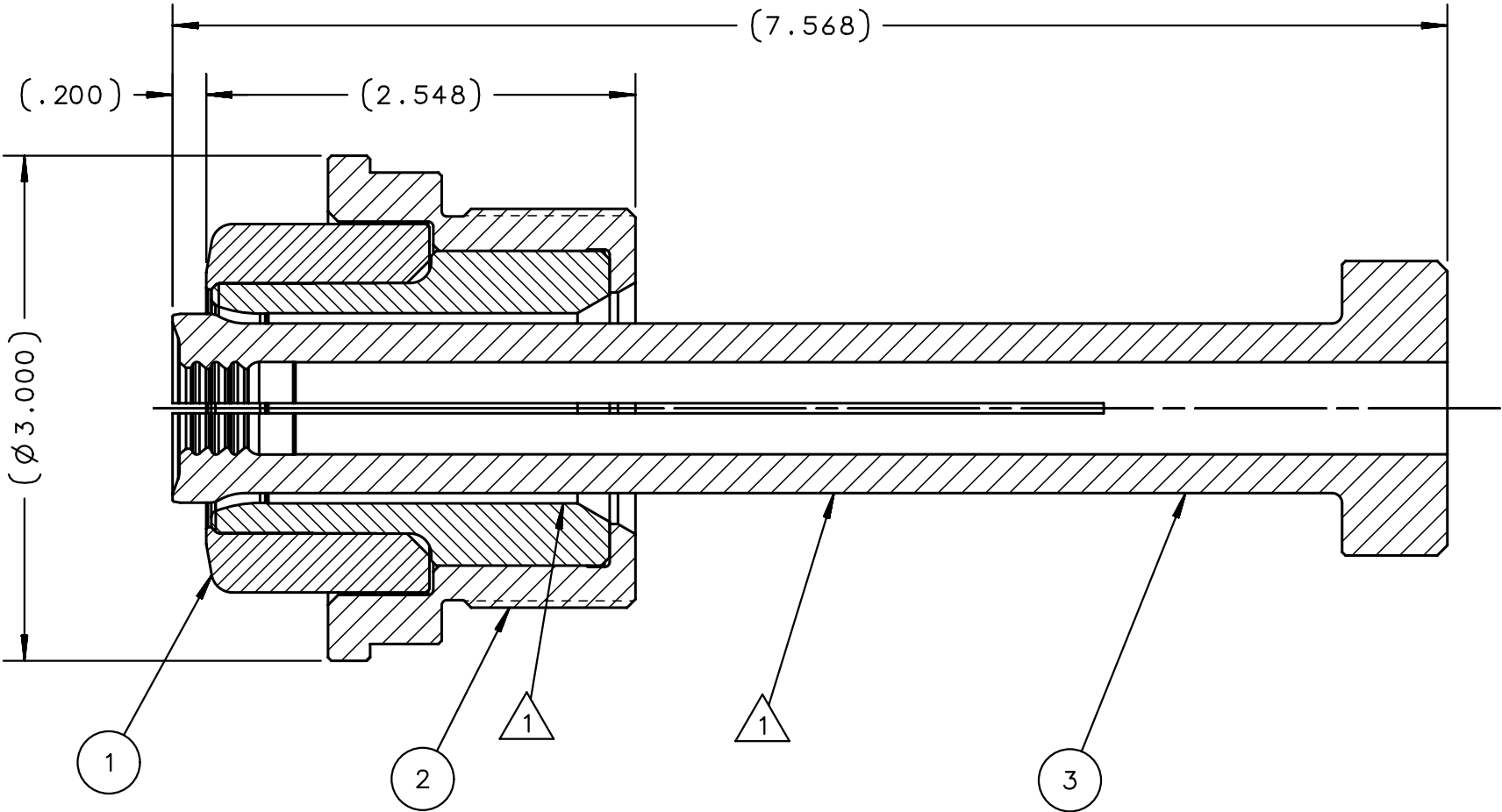
SECTION A-A
