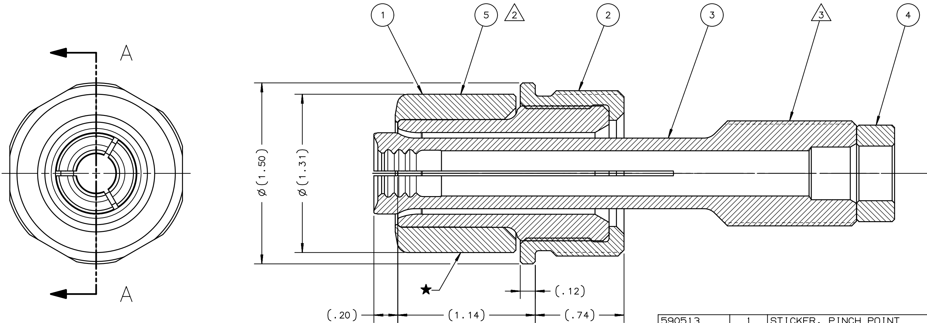
SECTION A-A
