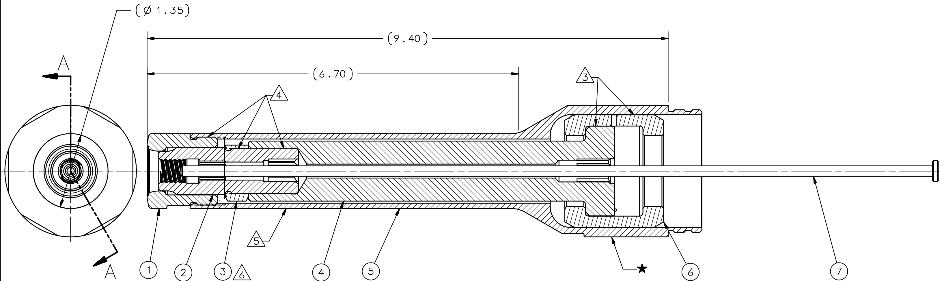
SECTION A-A
