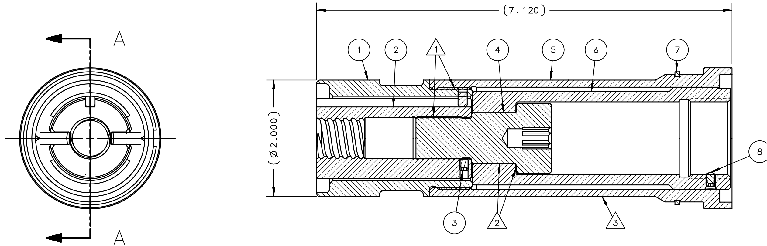
SECTION A-A
