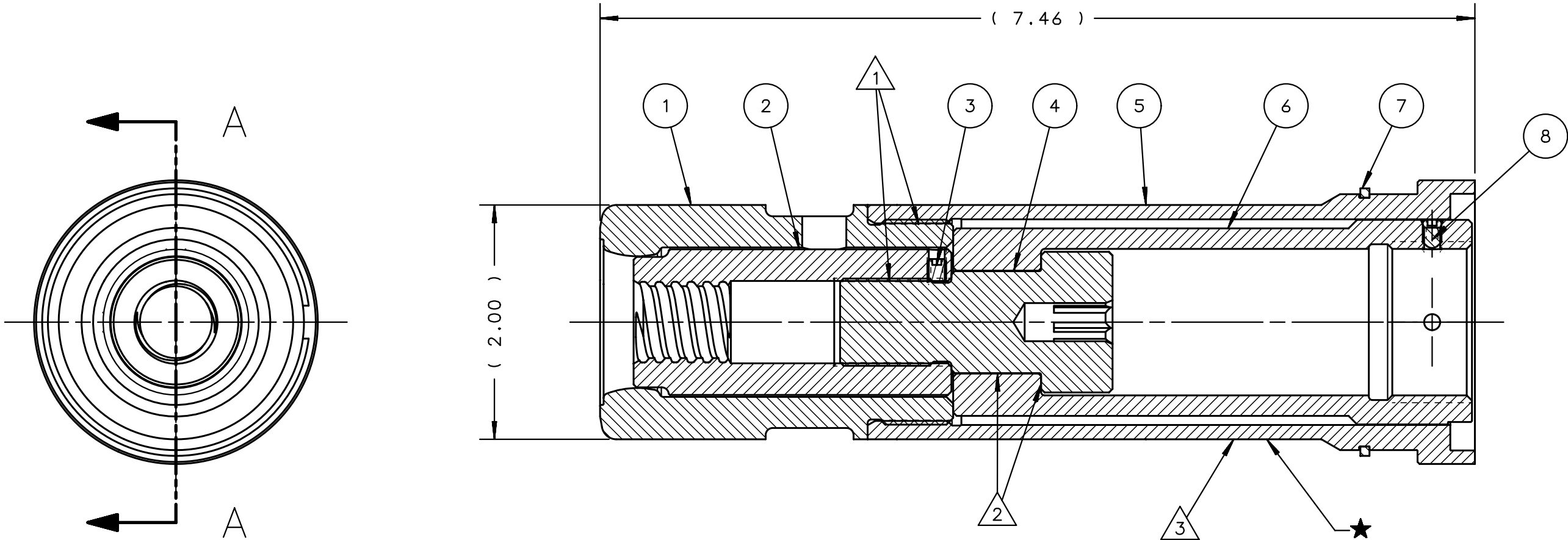
SECTION A-A
