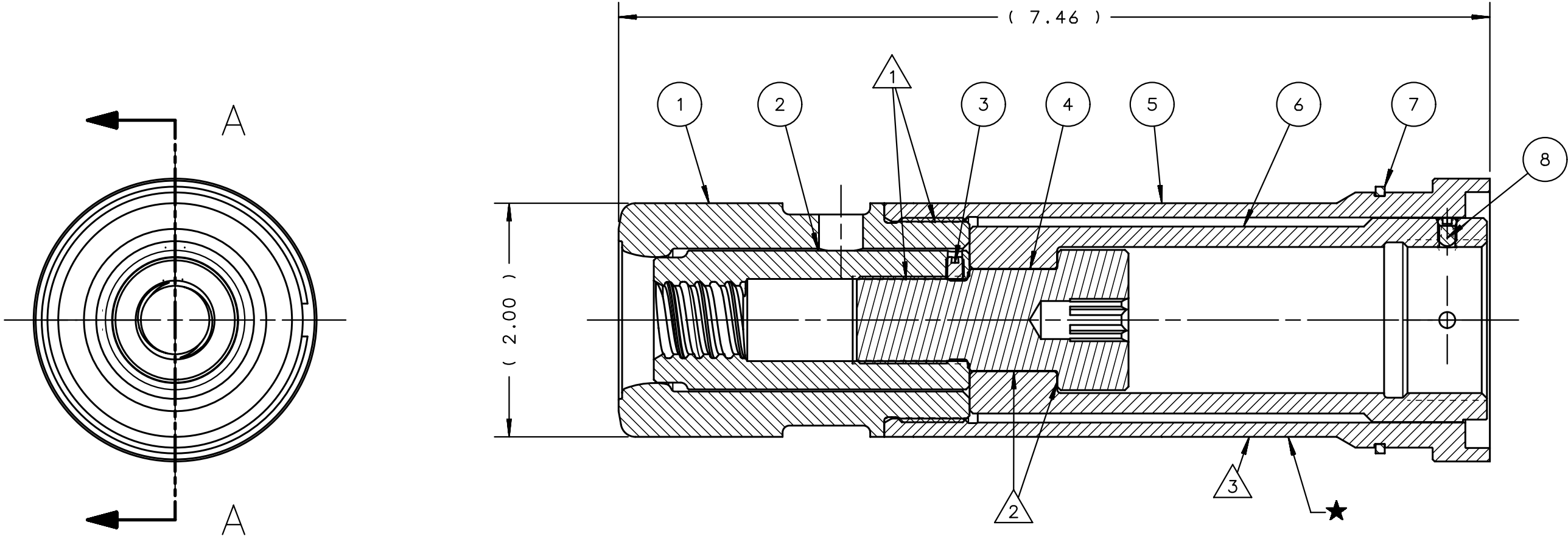
SECTION A-A
