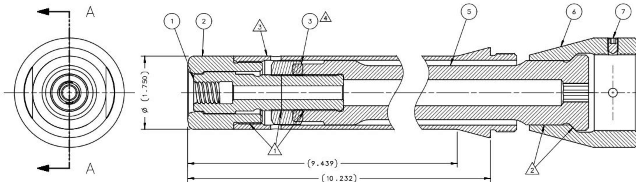
SECTION A-A
