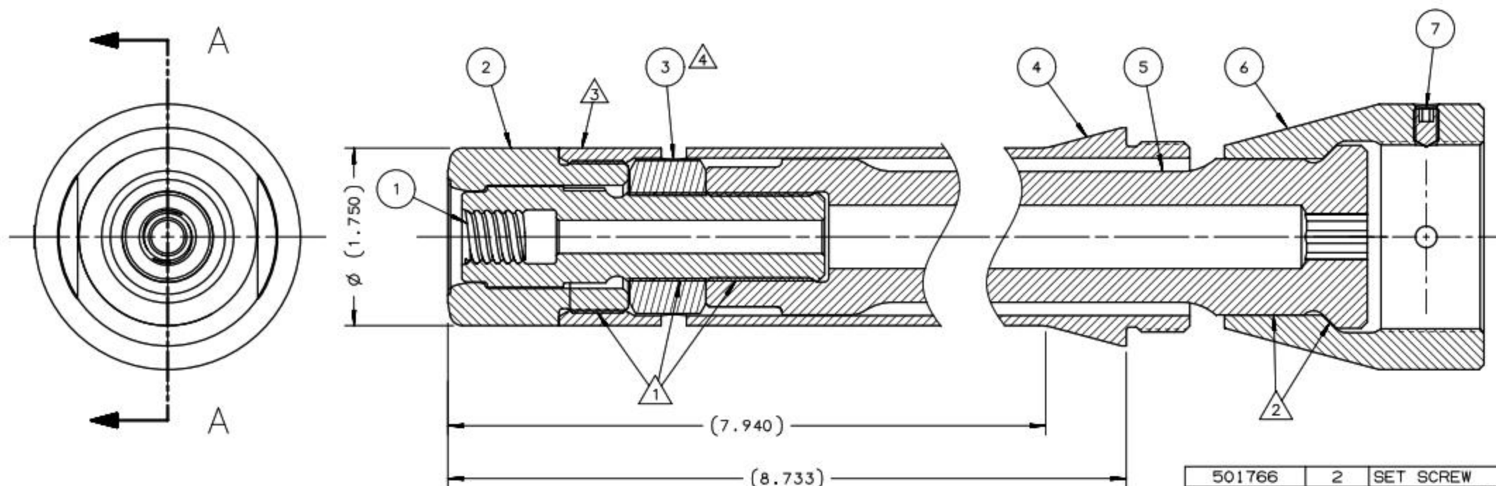
SECTION A-A
