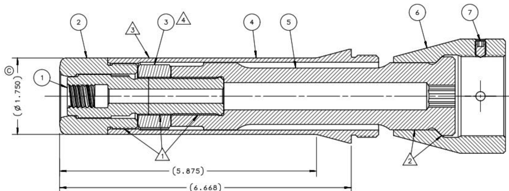
SECTION A-A
