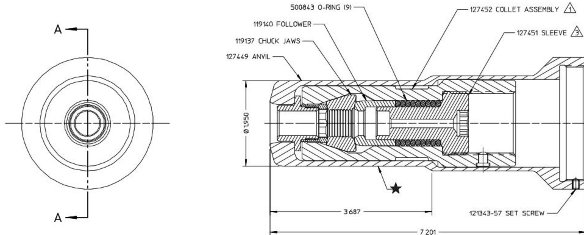
SECTION A-A
