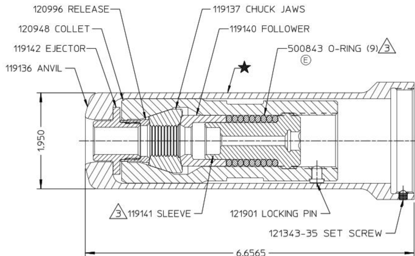
SECTION A-A
