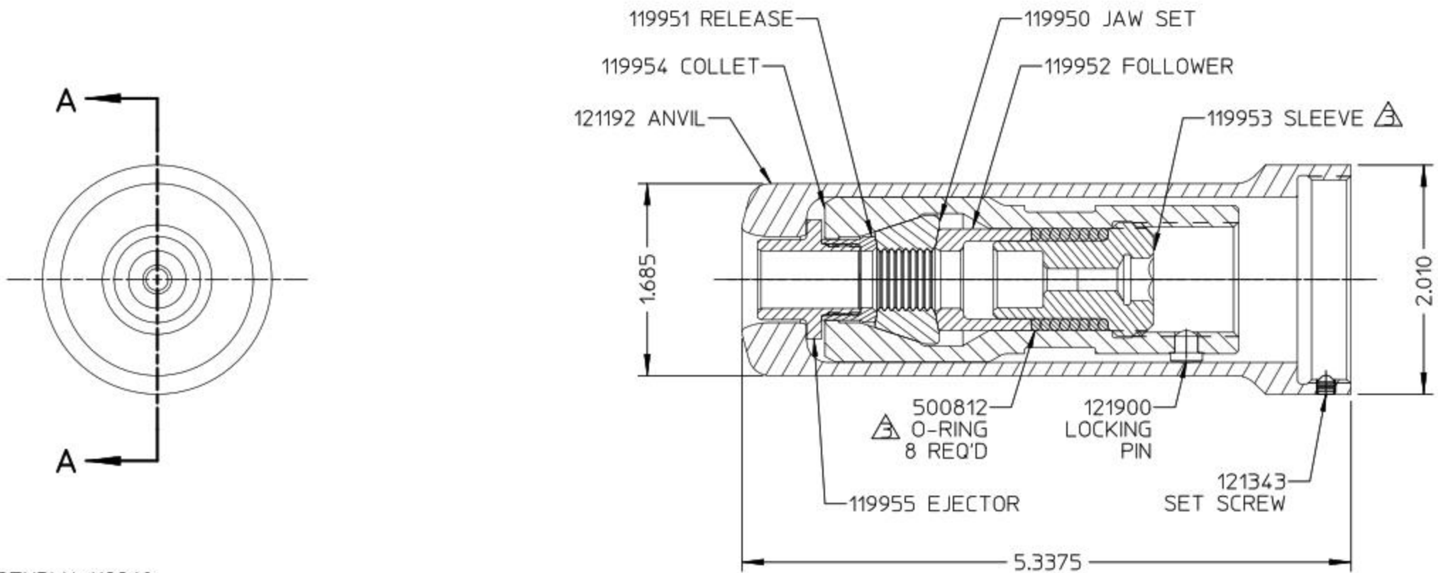
SECTION A-A
