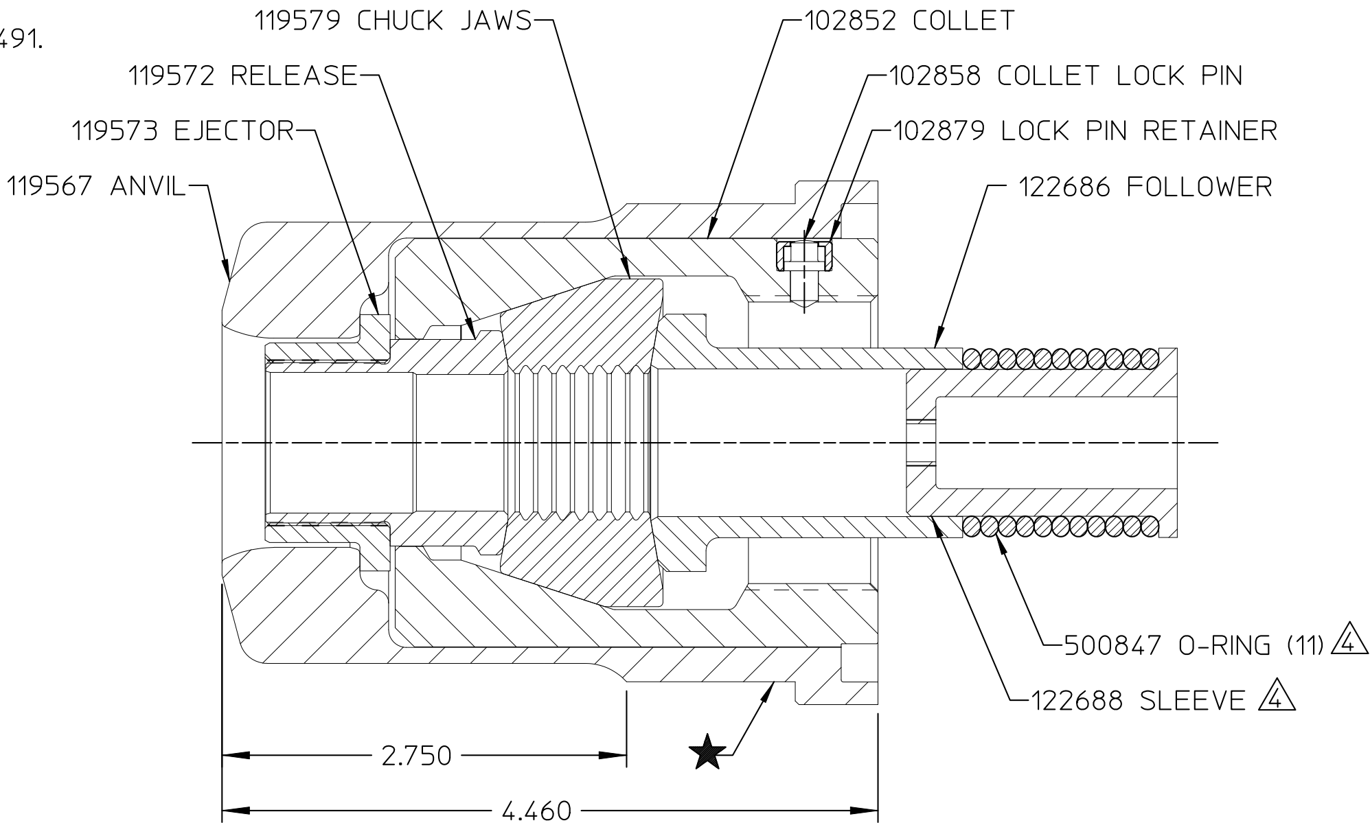
SECTION A-A
