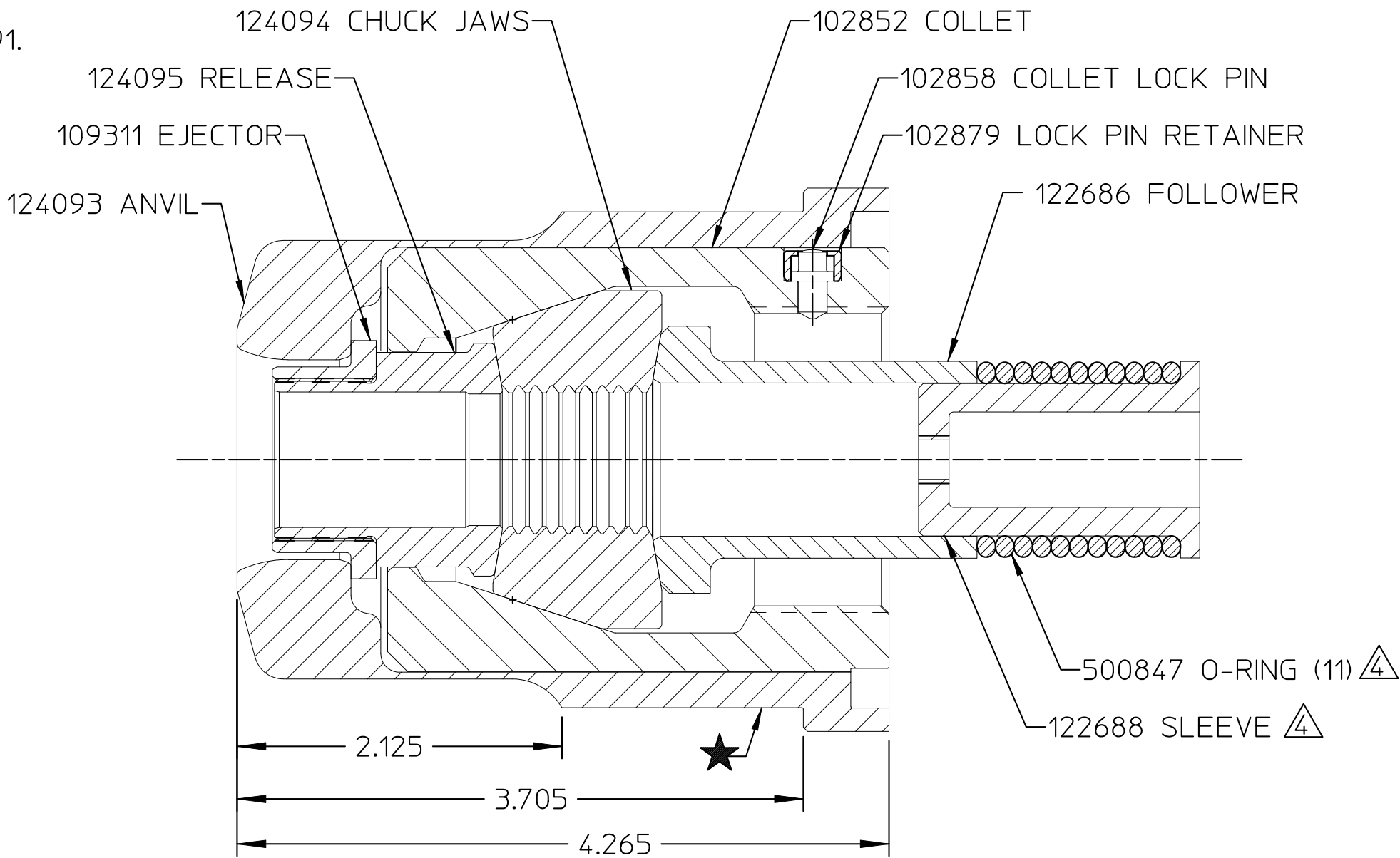
SECTION A-A
