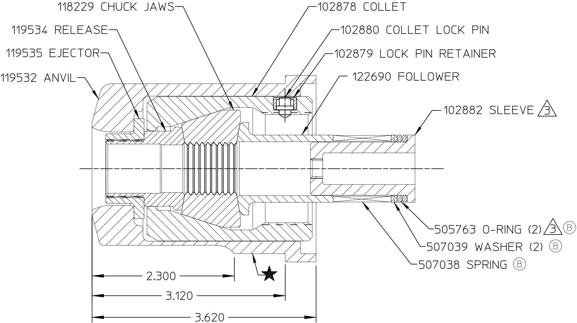
SECTION A-A
