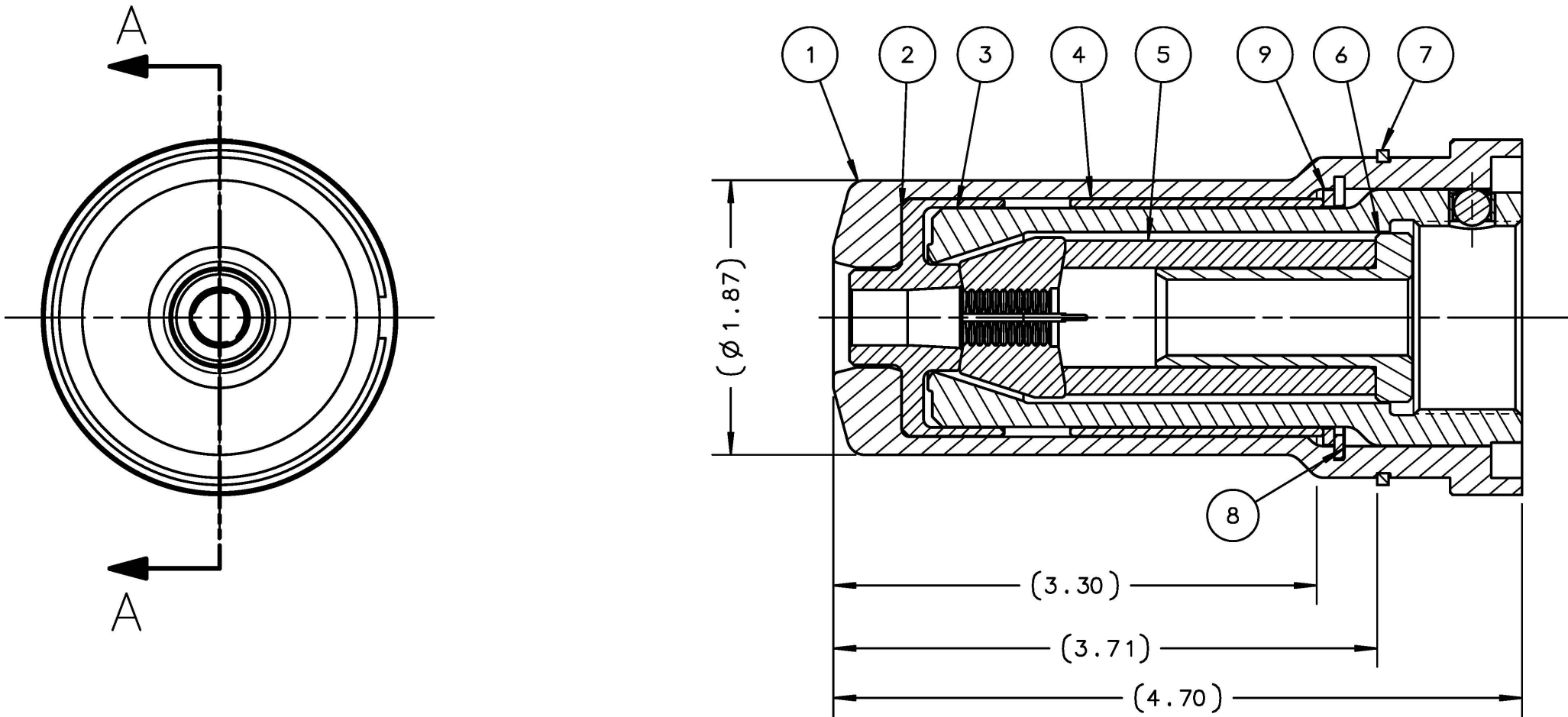
SECTION A-A
