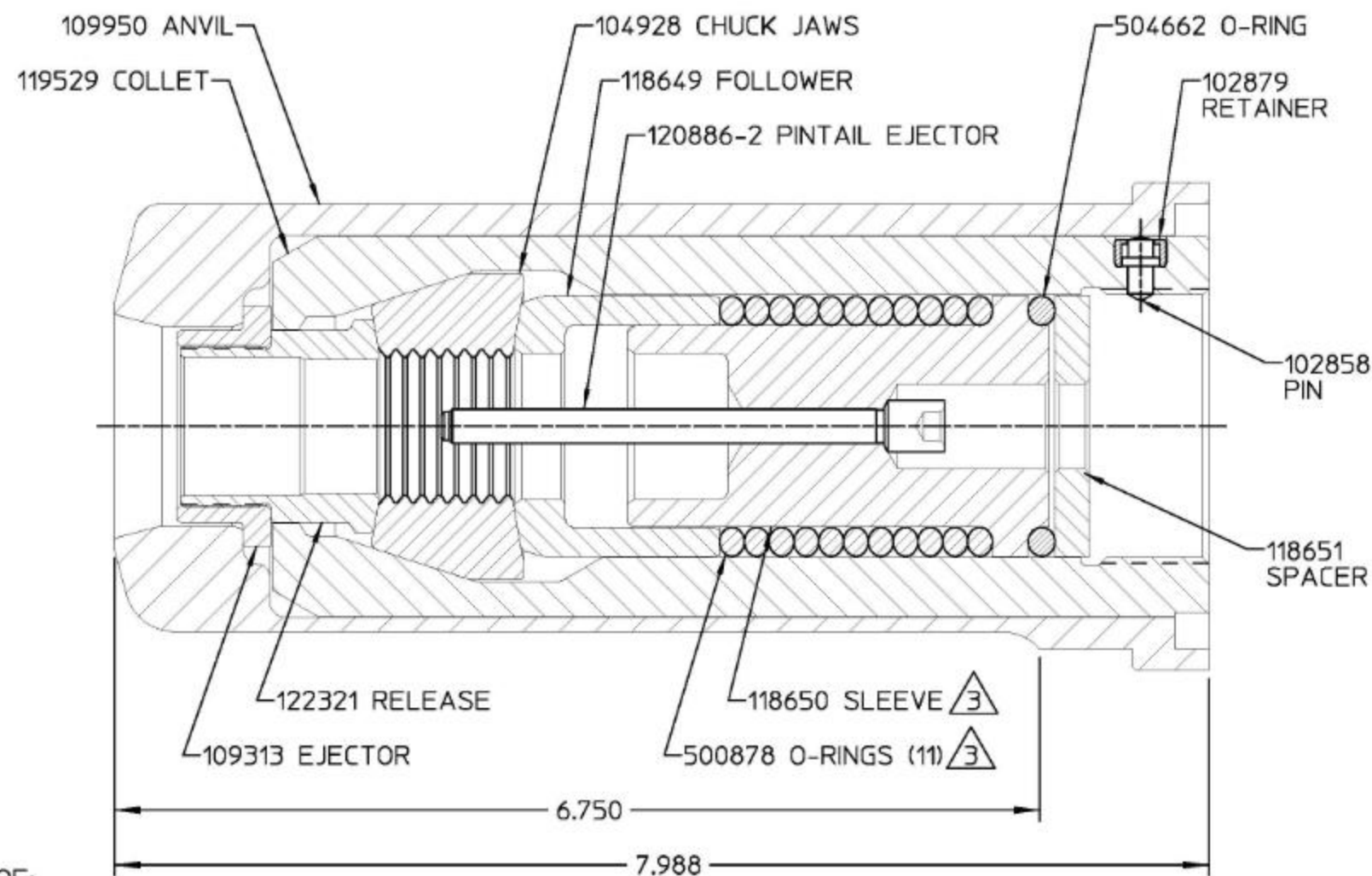
SECTION A-A
