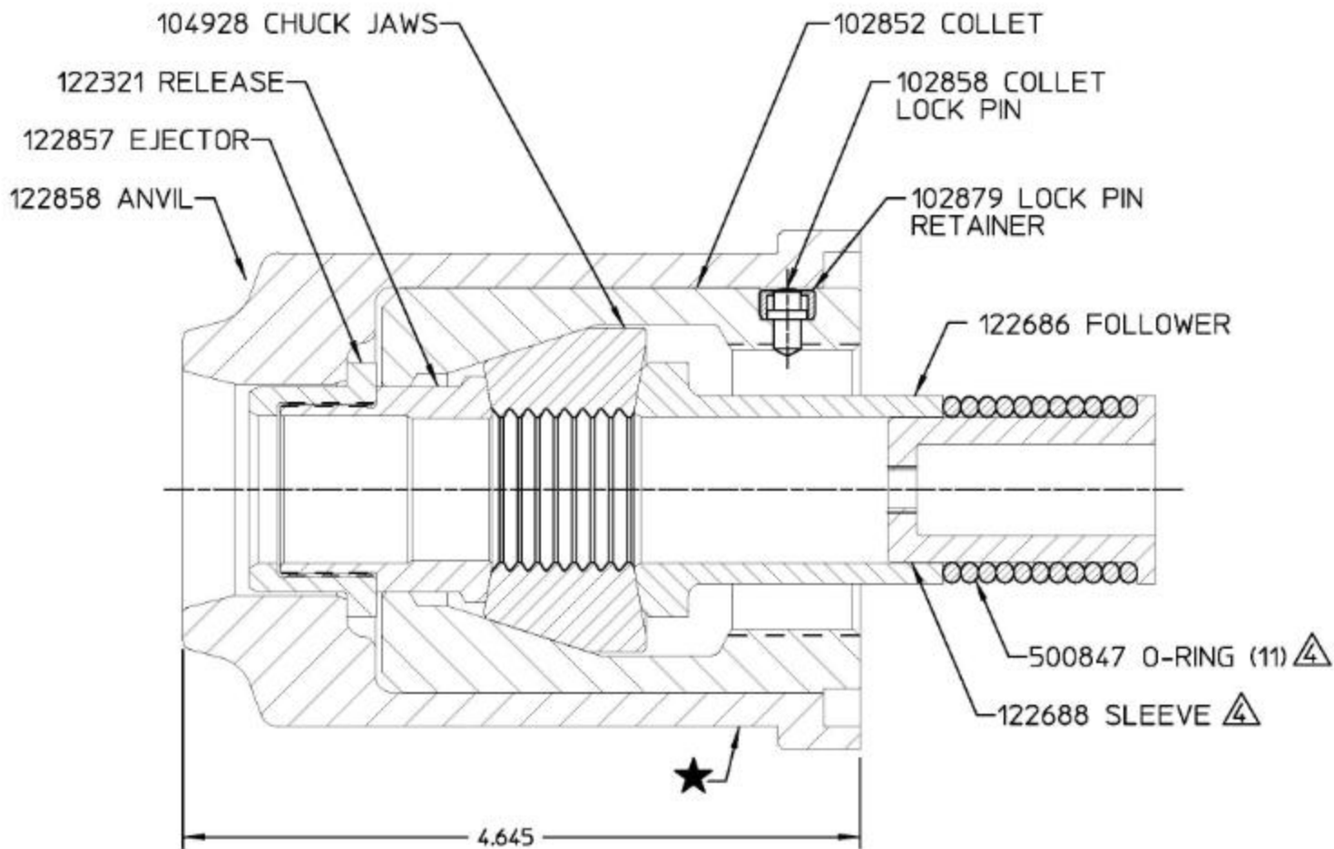
SECTION A-A
