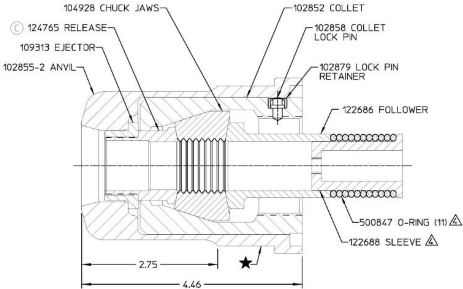
SECTION A-A
