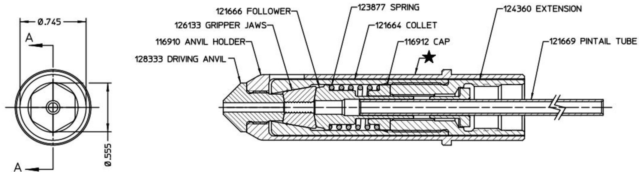
SECTION A-A
