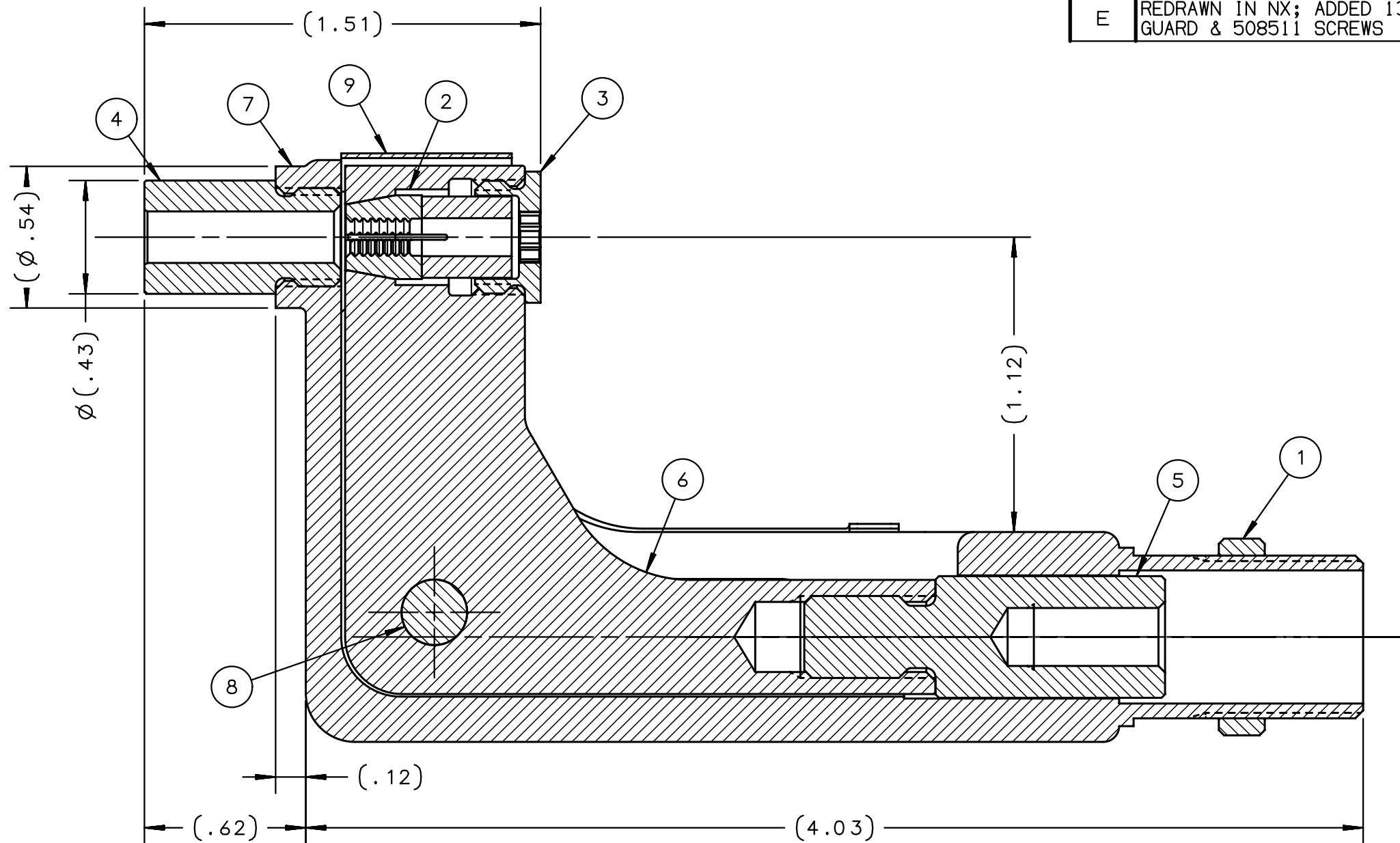
SECTION A-A
