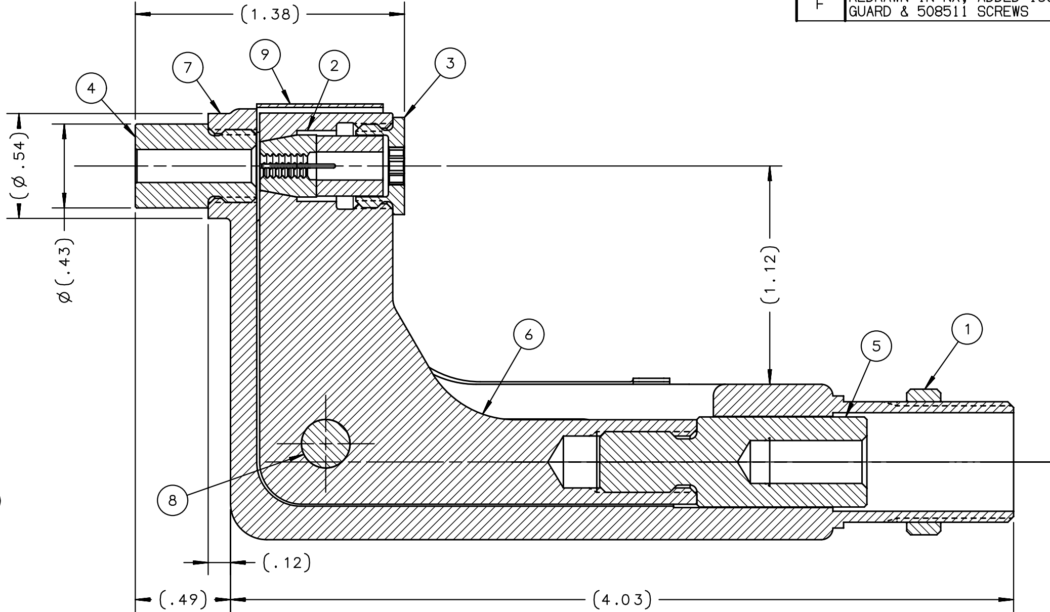
SECTION A-A
