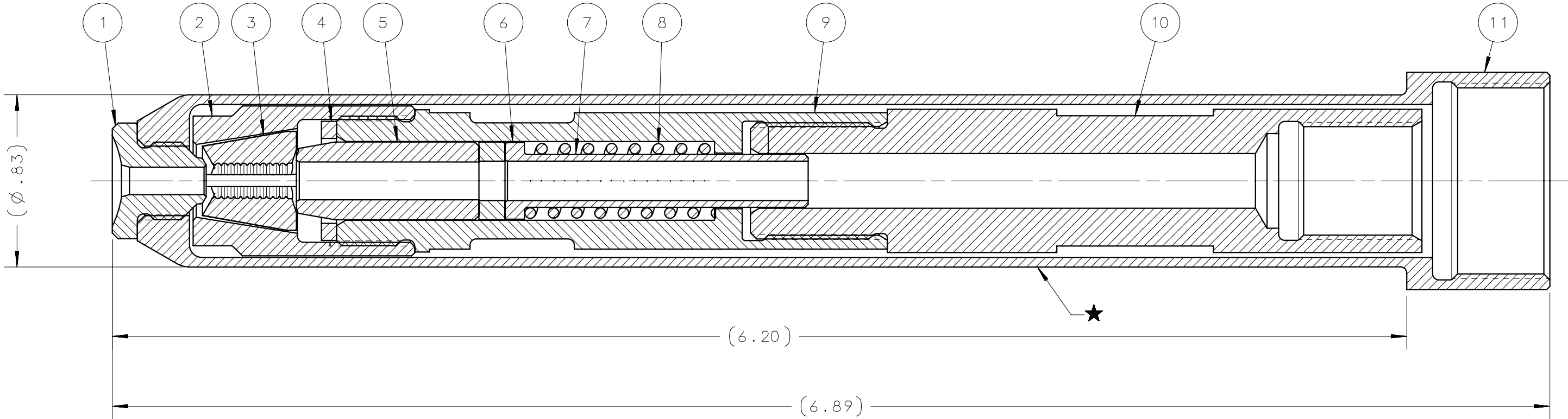
SECTION A-A
