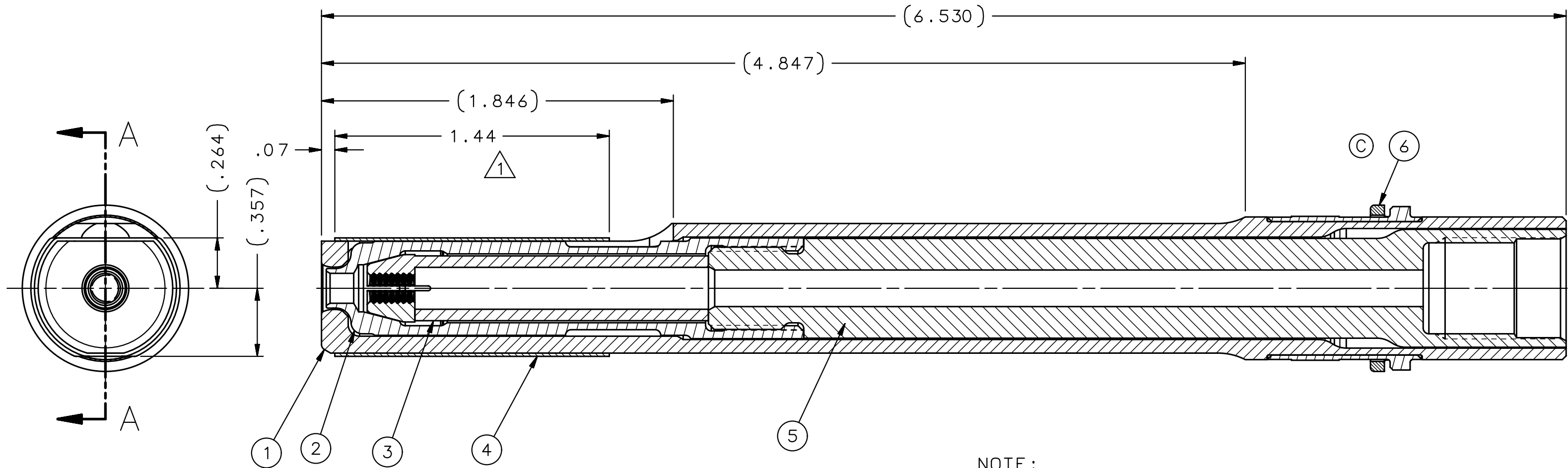
SECTION A-A
