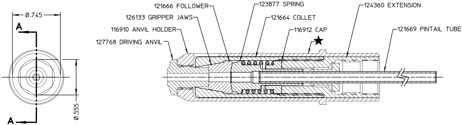
SECTION A-A
