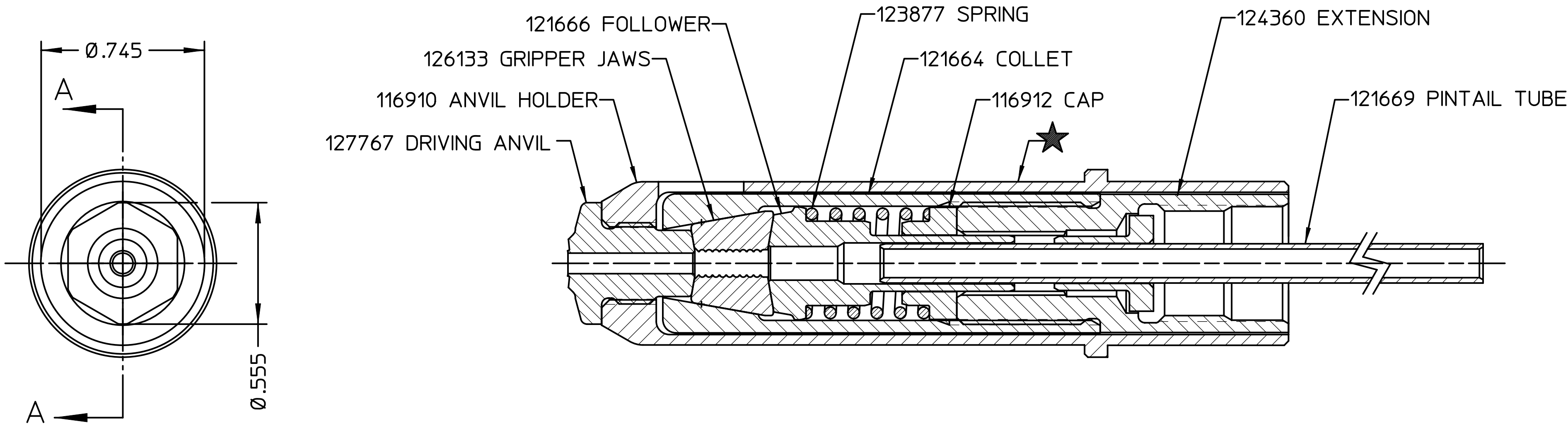
SECTION A-A
